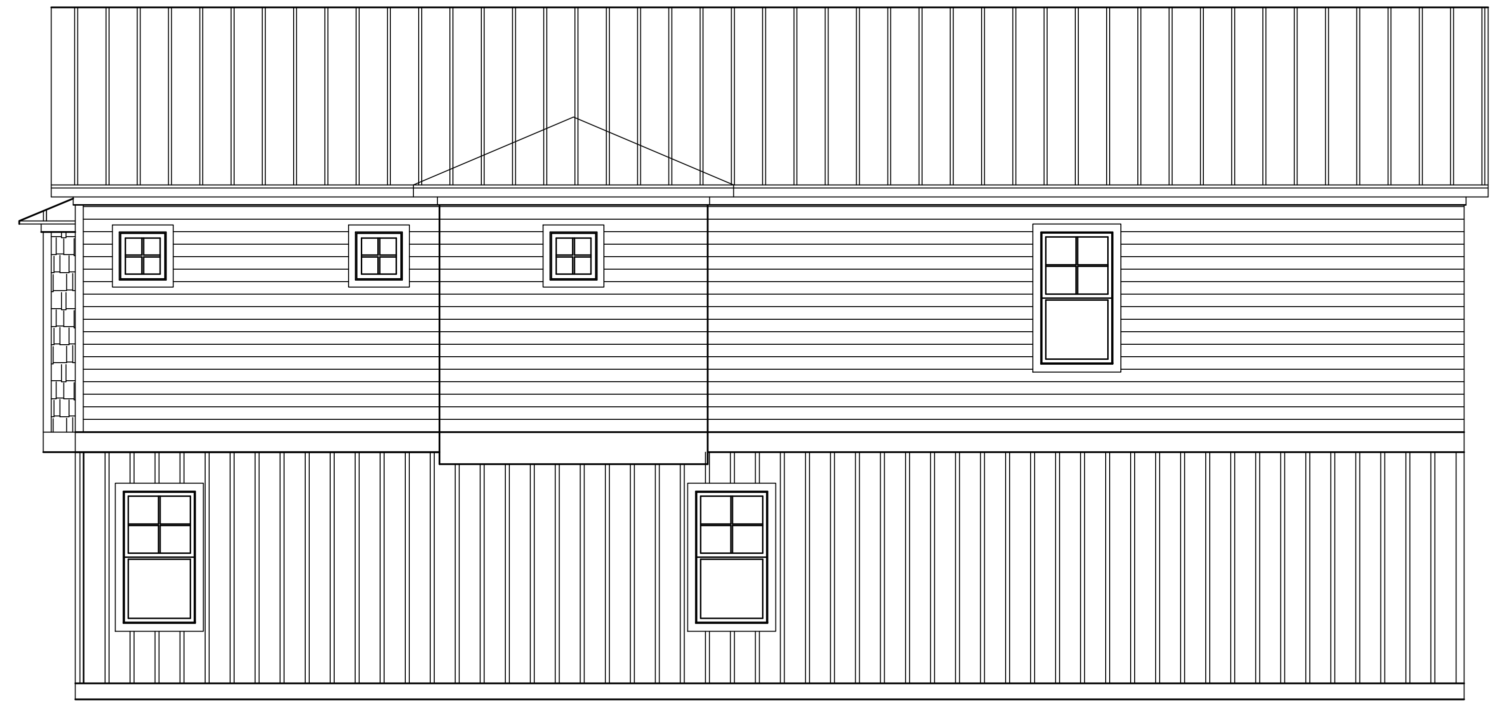
RIGHT ELEVATION
